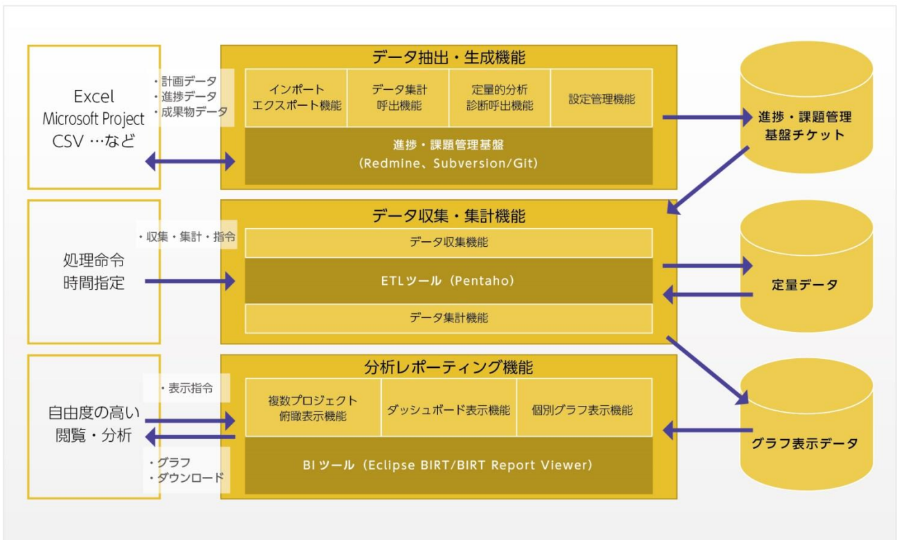
「EPM Base」構成図
